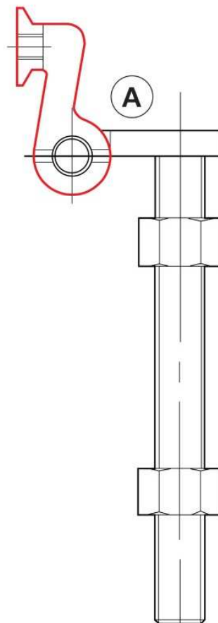
Spezialscharnier HSB Charnière spéciale HSB
