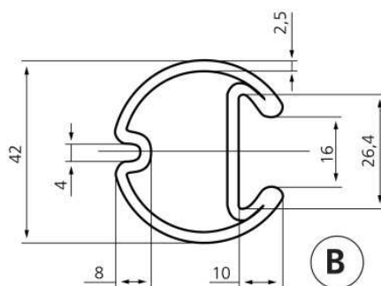
Sonderprofil HSB Profil spécial HSB
